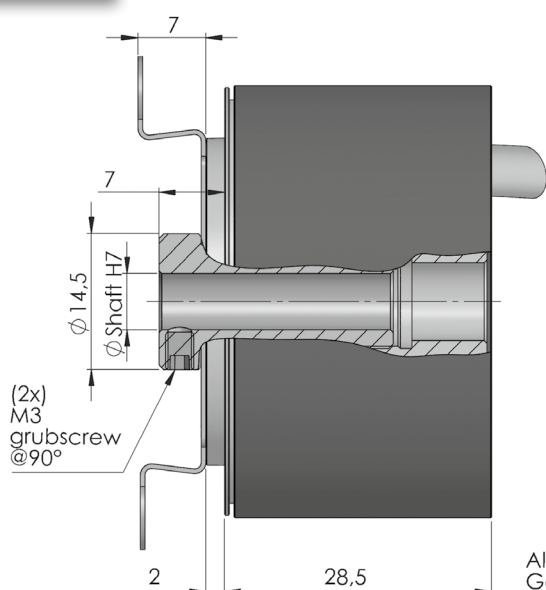
Flansch 2 / Flange 2
