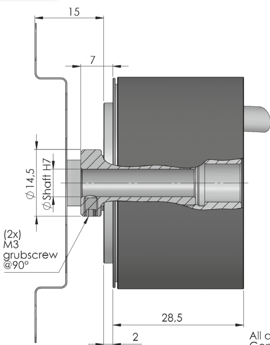
Flansch 3 / Flange 3
